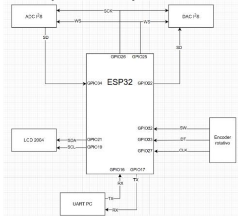
Fig. 1 diagrama en bloques
