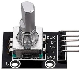
Fig. 5 encoder rotativo ky-040
